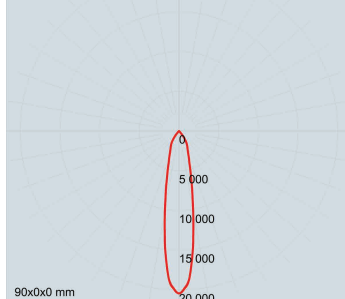
22° FWHM REFLECTOR
